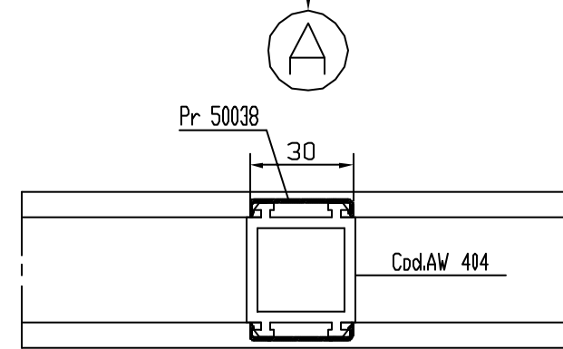
PARTICOLARE FRANCESINA
