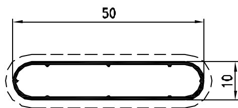
Pr. 50013 kg/m. 0.240
