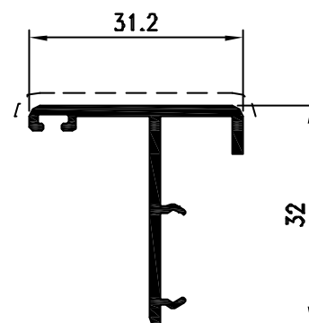
Pr. 50110 kg/m. 0.292
