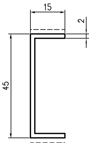
Pr 01060 kg/m. 0,383 sup.in vista mm. 30
