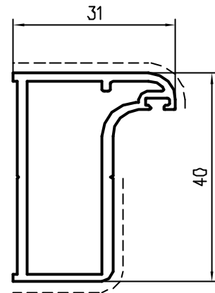
Pr 27388 kg/m. 0,618 sup.in vista mm. 74
