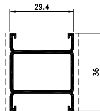
Pr. 50105 kg/m. 0.481
