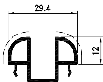
Pr. 50108 kg/m. 0.354
