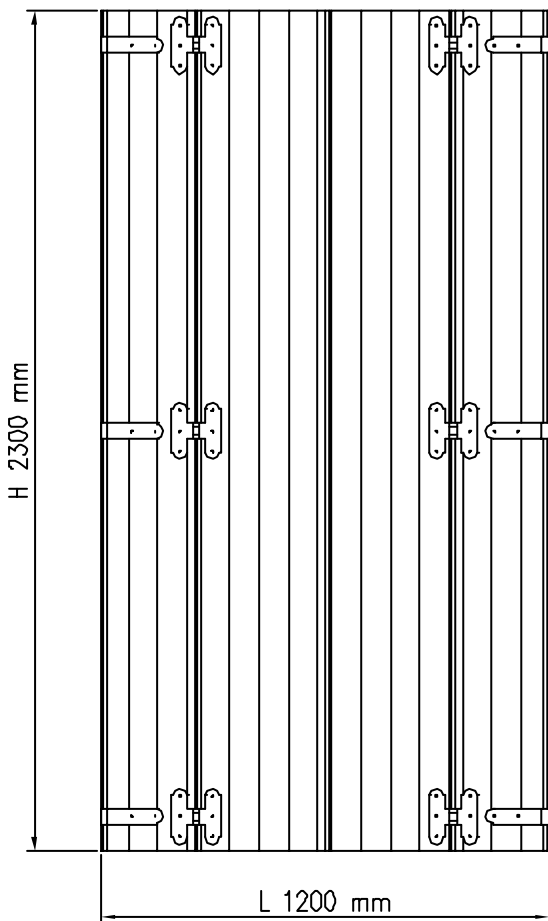
PROSPETTO ESTERNO
