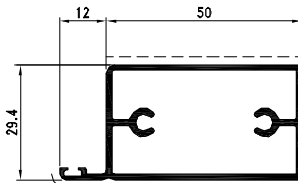
Pr. 50107 kg/m. 0.797
