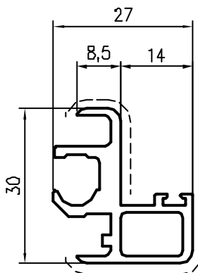
Pr 27393 kg/m. 0,556 sup.in vista mm. 62
