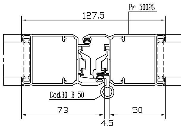
NODO PERSIANA A 3 ANTE
