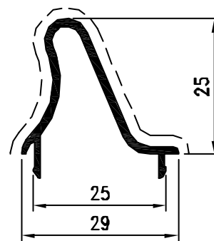
Pr. 50115 kg/m. 0.267
