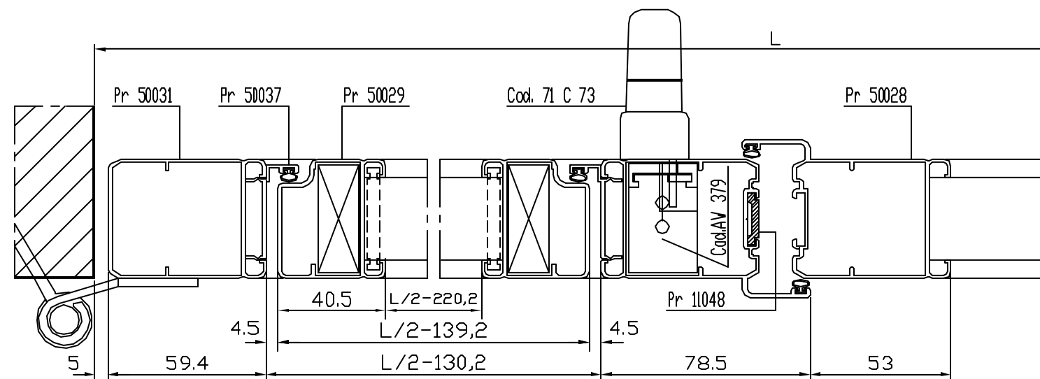
PARTICOLARE FRANCESINA
