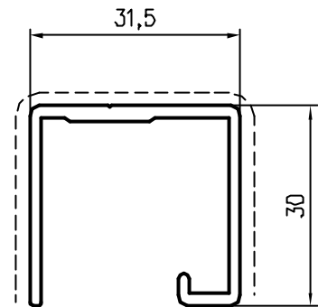
Pr 27388 kg/m. 0,618 sup.in vista mm. 74
