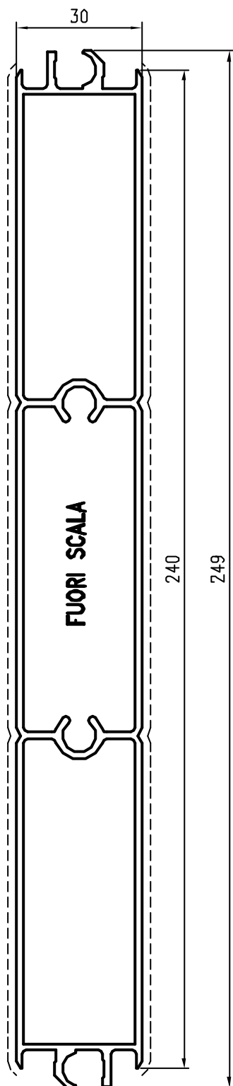
Pr 60154 kg/m. 2,884 sup.in vista mm. 480
