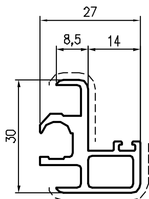
Pr 27385 kg/m. 0,548 sup.in vista mm. 62
