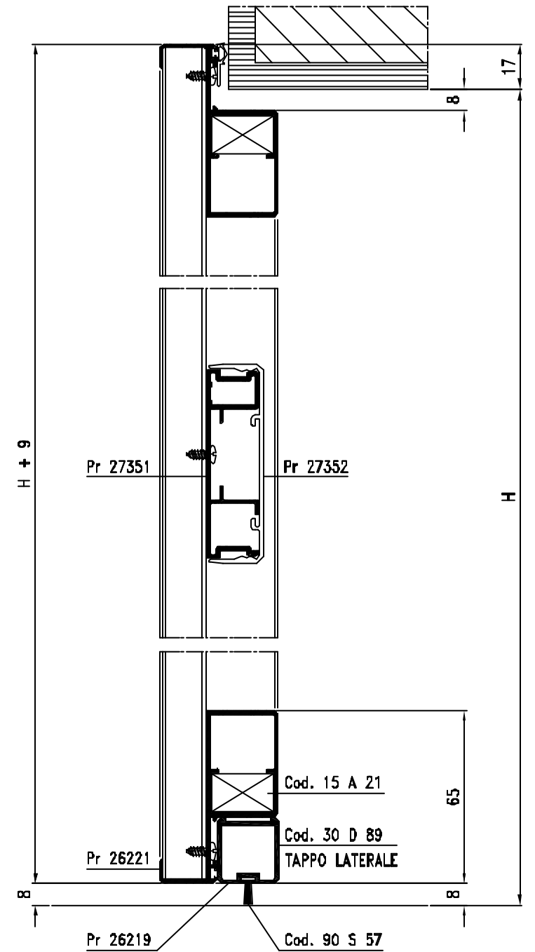
PORTA
