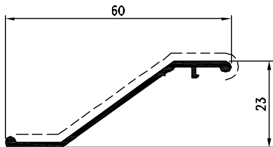
PROFILATO ALETTA FRANGISOLE
