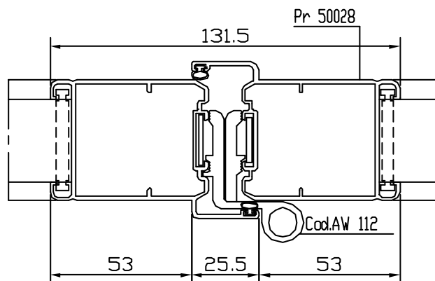
NODO PERSIANA A 3 ANTE
