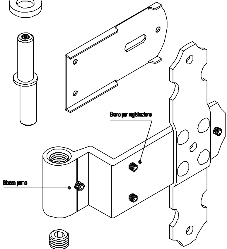
-1- Cardine da interno per pannello
