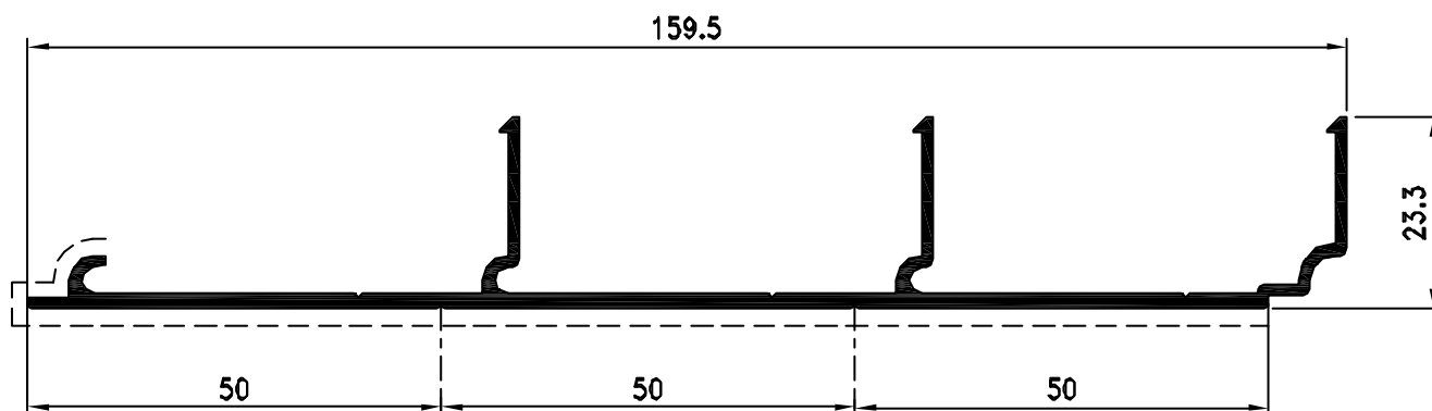
PROFILATO BASE MODULARE FRANGISOLE
