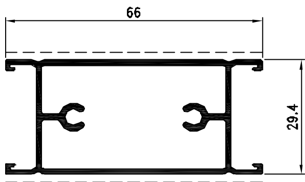
Pr. 50106 kg/m. 0.875
