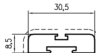
Pr 27390 kg/m. 0,567 sup.in vista mm. 42
