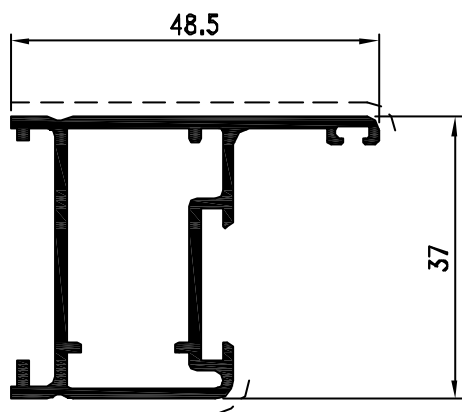
Pr. 50100 kg/m. 0.664
