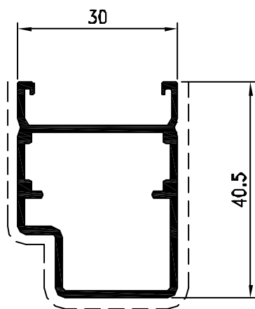
Pr. 50104 kg/m. 0.564
