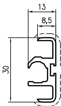
Pr 27384 kg/m. 0,343 sup.in vista mm. 42
