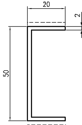
Pr 01081 kg/m. 0,464 sup.in vista mm. 40
