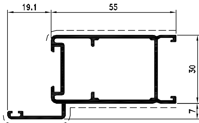
Pr. 50102 kg/m. 0.853
