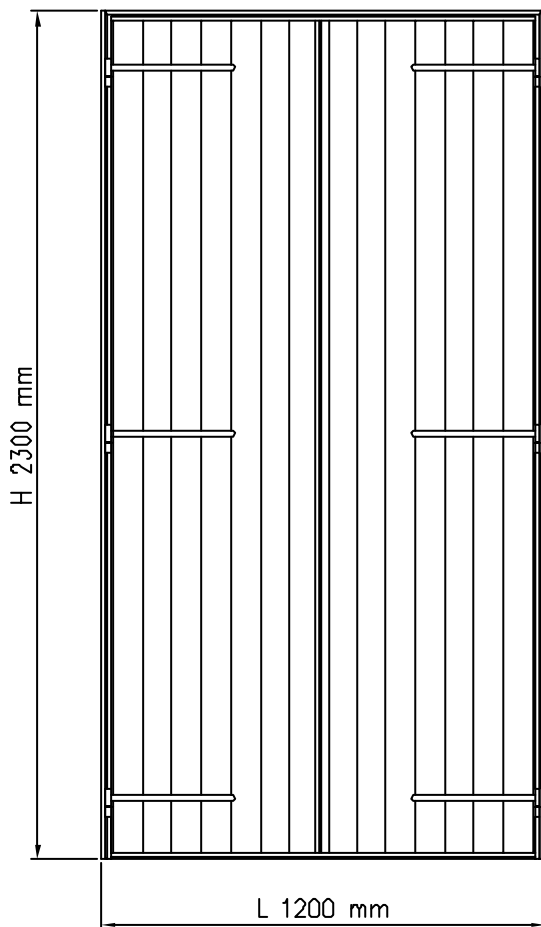
PROSPETTO ESTERNO
