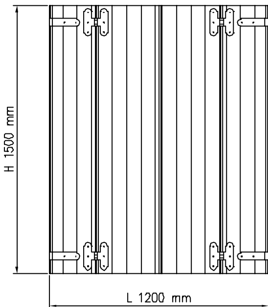
PROSPETTO ESTERNO
