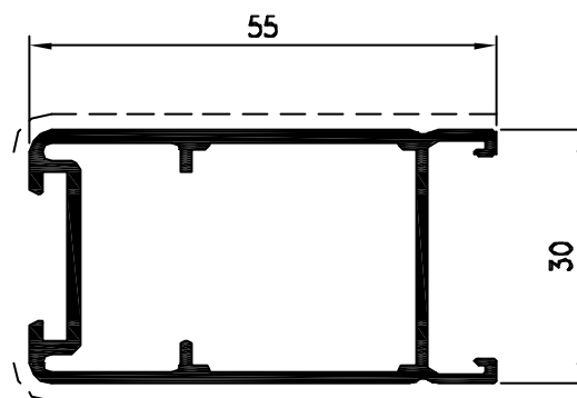
Pr. 50103 kg/m. 0.716
