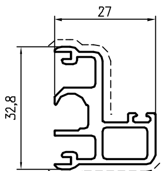
Pr 60156 kg/m. 0,618 sup.in vista mm. 71
