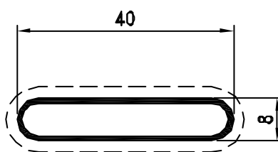
Pr. 50114 kg/m. 0.232
