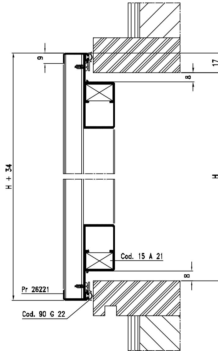
FINESTRA
