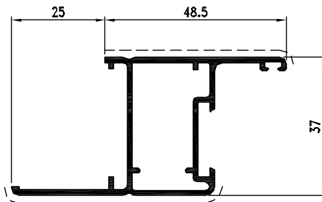
Pr. 50101 kg/m. 0.778
