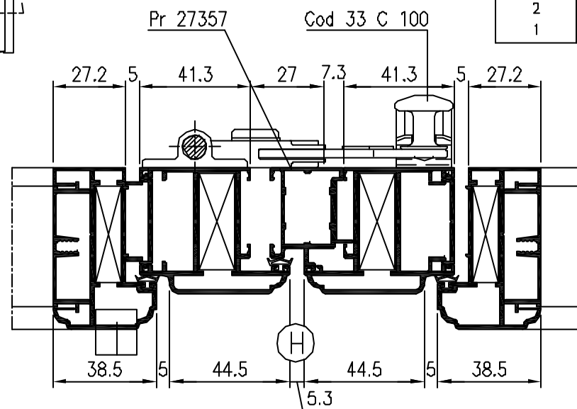
GELOSIA 2 ANTE
