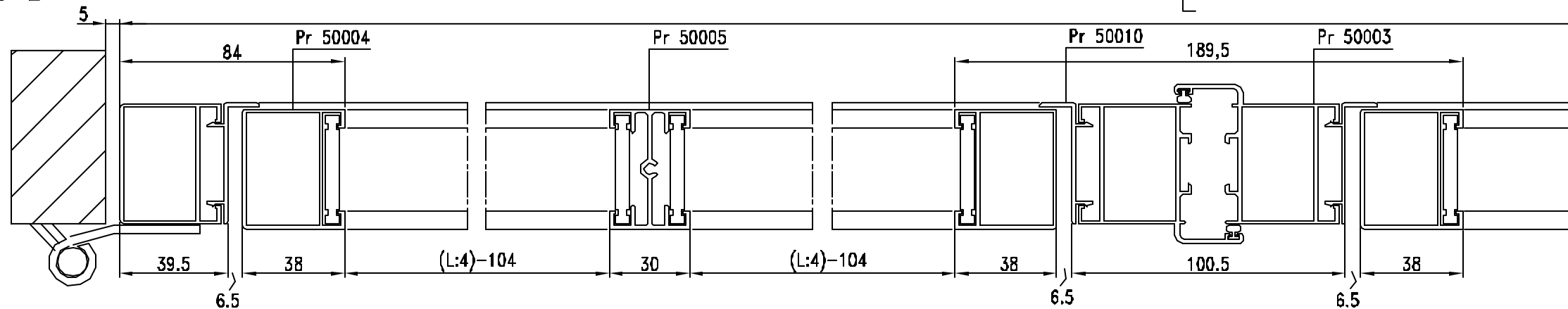
Sez. E-E
