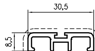
Pr 27459 kg/m. 0,292 sup.in vista mm. 42
