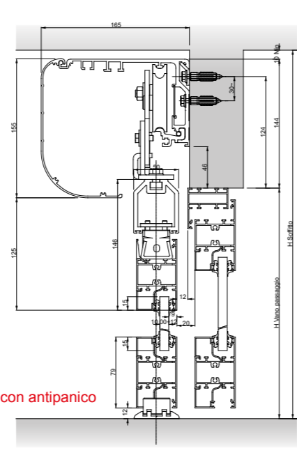
G38_Anta in vetro
