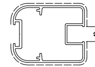
L-IT34642 sup.vista mm. 167 Kg./m 1.064
