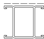
D0050105 kg/m. 0.481 Sup. in vista 74 TAPPO D00AW508
