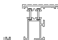
D1210618 sup.vista mm. 118 Kg./m 1.248
