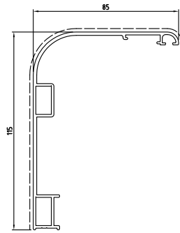
D3220112 sup.vista mm. 192 Kg./m 1.326
