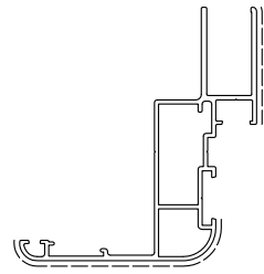
D3220079 sup.vista mm. 130 Kg./m 1.523
