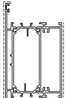
D1210865 Kg/m 2.613 Sup. in vista mm 225
