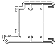
D3220093 sup.vista mm. 137 Kg./m 1.248
