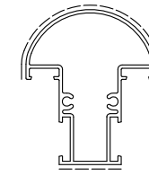
D3220090 sup.vista mm. 124 Kg./m 1.152
