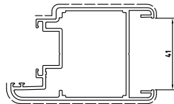
D3220092 sup.vista mm. 171 Kg./m 1.458
