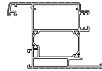
D1210889 Kg/m 2.621 Sup. in vista mm 210 TAPPO EST. D4240304 TAPPO INT. D4240166
