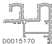
D0015170 sup.vista mm. 95 Kg/m 1.149
