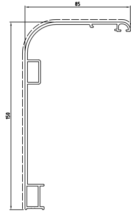
D3220141 sup.vista mm. 227 Kg./m 1.538
