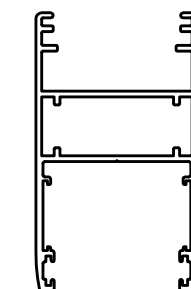
D3240053 Lg 6650
