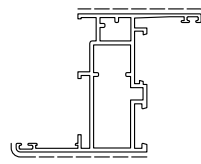
D3210287 sup.vista mm. 109 Kg./m 1.134
