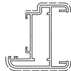
D3220094 sup.vista mm. 105 Kg./m 0.994
