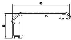
D3220106 sup.vista mm. 114 Kg./m 0.810
