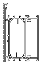
D1210865 Kg/m 2.613 Sup. in vista mm 225
