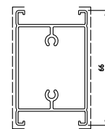
D0050043 sup.vista mm. 151 kg/m 0.988
