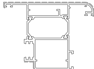
D1210837 Kg/m 2.088 Sup. in vista mm 178
