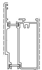
D1210604 sup.vista mm. 141 Kg./m 1.694
