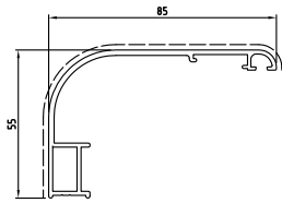
D3220109 sup.vista mm. 132 Kg./m 0.876
