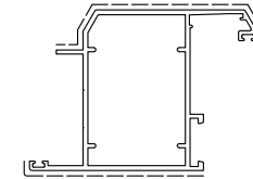
D0024463 sup.vista mm. 163 kg/m 1.336 TAPPO D0013D60
