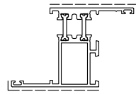
D1210501 sup.vista mm. 108 Kg./m 1.100
