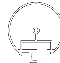
D3270019 sup.vista mm. 159 Kg./m 1.350 TAPPO D020D100
