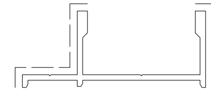
D3290163 sup.vista mm. 63 Kg./m 0.413
