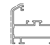
D3210070 sup.vista mm. 117 Kg/m 1.072
