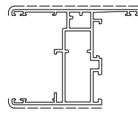
D3210299 sup.vista mm. 136 Kg./m 1.256
