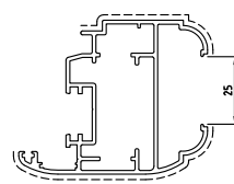
D3210201 sup.vista mm. 145 Kg./m 1.269 TAPPO D4240126
