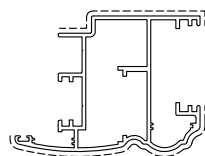
D3260057 sup.vista mm. 161 Kg./m 1.338 TAPPO D4240012
