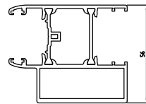
D1074052 kg/m. 1.625 sup. in vista mm. 190 TAPPO D4074006
