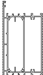
D1210861 Kg/m 3.293 Sup. in vista mm 285
