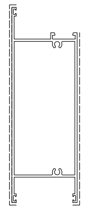
D3220020 sup.vista mm. 298 kg/m 2.014
