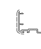
D0026261 sup.vista mm. 35 Kg./m 0.305
