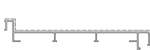
D3290066 sup.vista mm. 224 Kg./m 1.291 TAPPO D6240015
