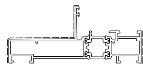
D1210302 sup.vista mm. 131 Kg./m 1.676
