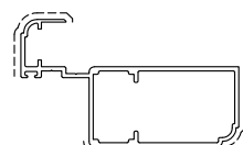
D3260044 sup.vista mm. 120 Kg./m 0.972
