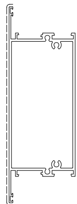
D3210295 sup.vista mm. 236 Kg./m 2.403
