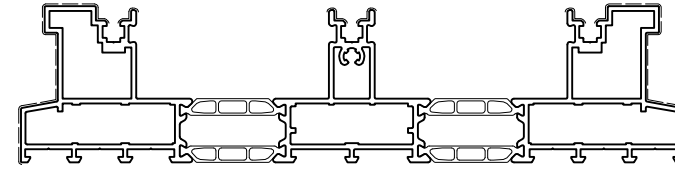
SC9K030 sup.vista mm. 000 Kg./m 5.192
