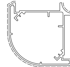
D0024499 sup.vista mm. 174 Kg./m 2.031
