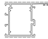
D3210290 sup.vista mm. 127 Kg./m 1.342
