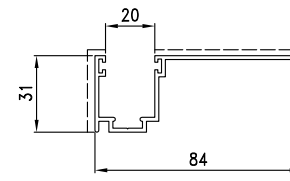
D3290160 sup.vista mm. 134.8 Kg./m 0.815
