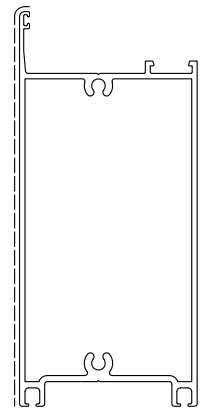
D3220004 sup.vista mm. 303 Kg./m 3.086
