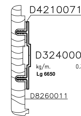
D3240053 Lg 6650
