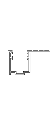
D3290111 sup.vista mm. 95 Kg./m 0.653
