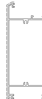
D0024469 sup.vista mm. 292 kg/m 2.238
