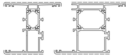
D1211006 kg/m. 1.477 sup. in vista mm. 135
