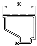
SGC 2330 sup.vista mm. 000 Kg./m 0.341
