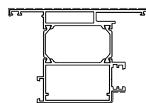
D1210881 Kg/m 2.455 Sup. in vista mm 202 TAPPO EST. D4240166 TAPPO INT. D4240304
