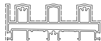
D0015177 sup.vista mm. 30 Kg/m 2.764
