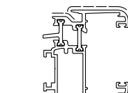
D1210674 sup.vista mm. 132 Kg./m 1.399
