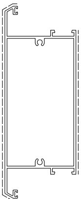
D0024468 sup.vista mm. 294 kg/m 2.218
