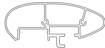
D3270013 sup.vista mm. 183 Kg./m 1.731 TAPPO DX D020D103 TAPPO SX D020D104
