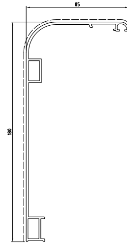
D0034761 sup.vista mm. 258 Kg./m 1.703
