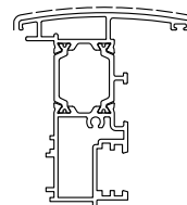
D1210007 kg/m. 1.502 sup. in vista mm. 85 TAPPO D4240101
