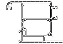
D1210891 Kg/m 2.614 Sup. in vista mm 208 TAPPO EST. D4240304 TAPPO INT. D4240166
