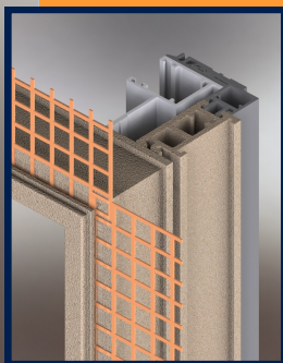
Soluzione modulare con guida per avvolgibile
