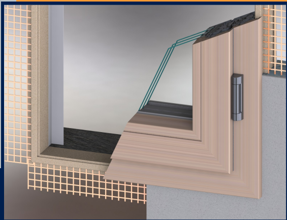
Dettagli di posa (INTERNO)
