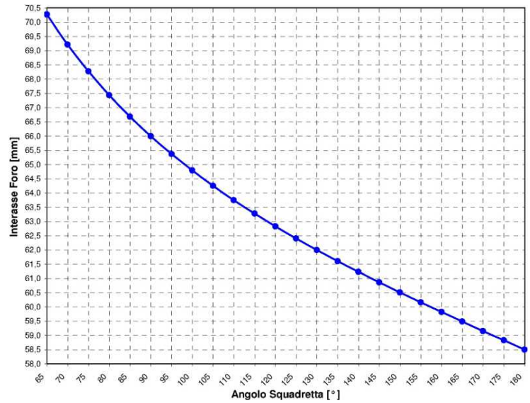
Interasse foratura D4250134
