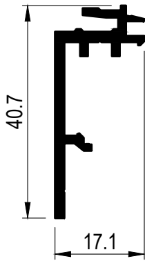
W4000187 | Profilo perforato
