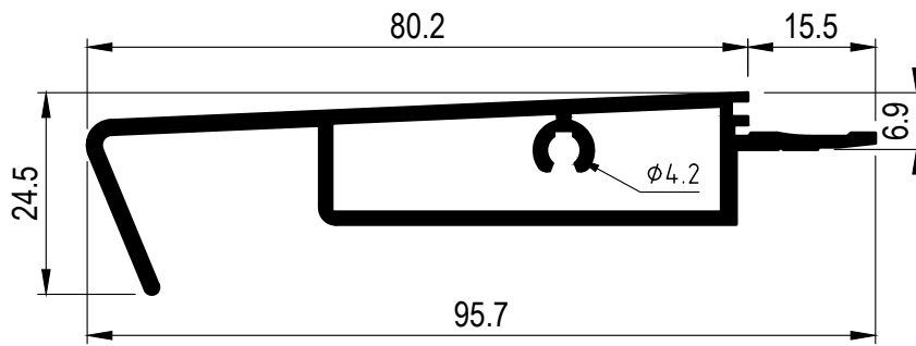
W4000185 | Profilo preforato. Tappo 4040455
