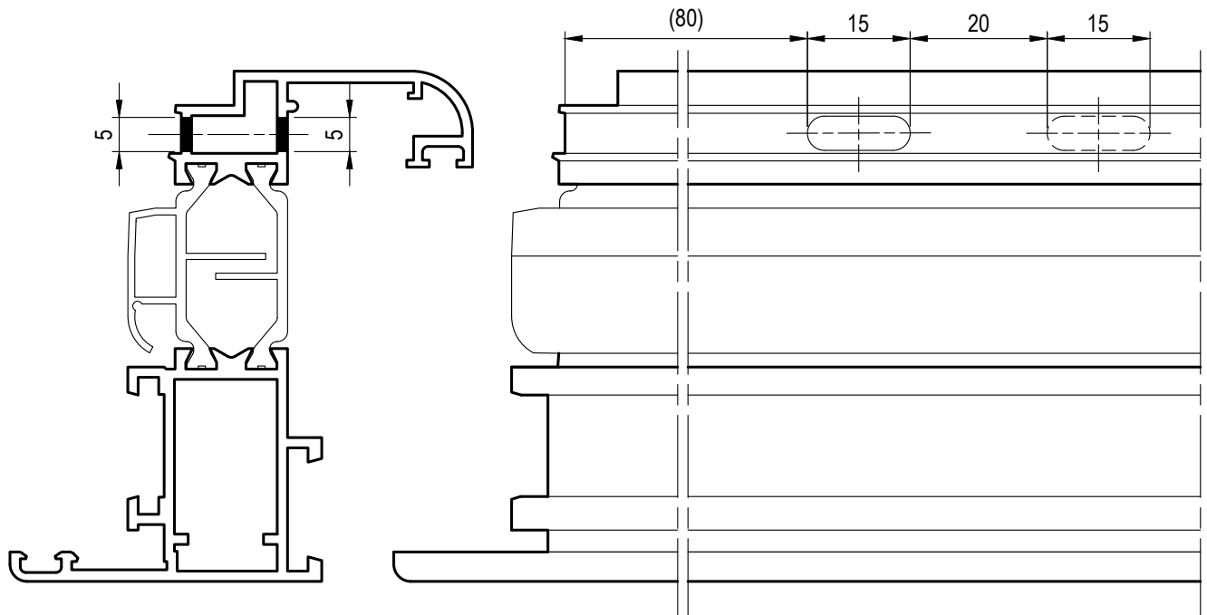
Schema lavorazione
