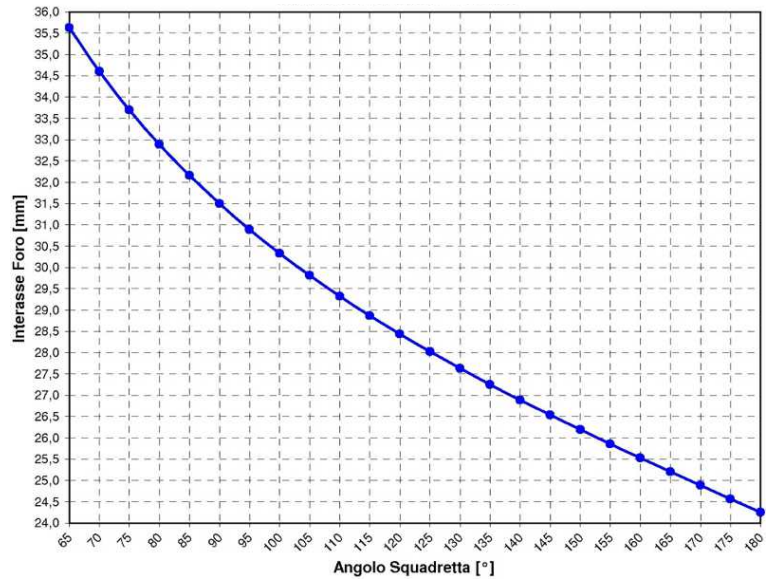
Interasse foratura D4250135
