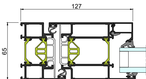
PORTA SOLEAL NEXT 65 sezione laterale
