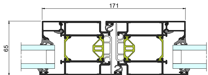
PORTA SOLEAL NEXT 65 sezione centrale
