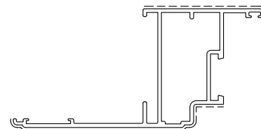
D3260264 kg/m. 0.946 sup. in vista mm. 139
