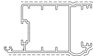
D3260018 Kg./m 1.172 sup.vista mm. 163 TAPPO D4240071
