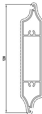
D0027494 sup.vista mm. 259 Kg./m 1.173
