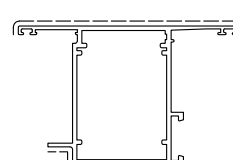
D3220069 sup.vista mm. 156 Kg./m 1.301 TAPPO D0015D30
