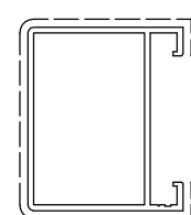
D0050004 sup.vista mm. 135 Kg./m 0.653 TAPPO D00AW042
