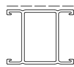
D0050105 kg/m. 0.481 Sup. in vista 74 TAPPO D00AW508
