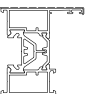
SC9V152 sup. vista mm. 116 Kg./m 1.829
