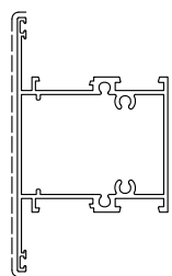
D3210294 sup.vista mm. 96 Kg./m 1.391
