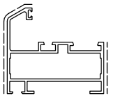
D3210071 sup.vista mm. 93 Kg/m 0.964
