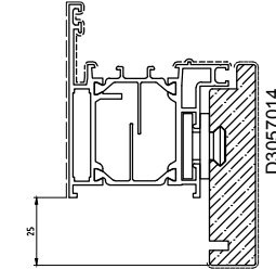
D1057053 Kg/m 1.564 Sup. in vista mm 76
