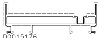
D0015176 sup.vista mm. 95 Kg/m 1.828
