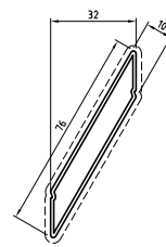
D3260224 sup.vista mm. 160 Kg./m 0.505
