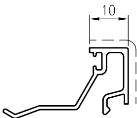
D3290101 sup.vista mm. 24.5 Kg./m 0.210
