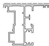
D3210293 sup.vista mm. 81 Kg./m 1.185 TAPPO EST. D4240023 TAPPO INT. D4240025
