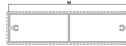
D3260227 sup.vista mm. 400 Kg./m 2.168
