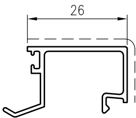
D3290105 sup.vista mm. 40.5 Kg./m 0.231
