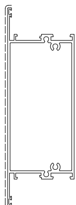
D3210295 sup.vista mm. 236 Kg./m 2.403
