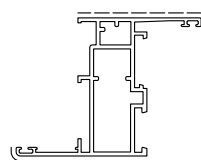
D3210287 sup.vista mm. 109 Kg./m 1.134
