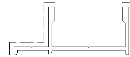
D3290163 sup.vista mm. 63 Kg./m 0.413
