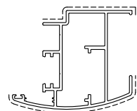
D0060908 sup.vista mm. 139 Kg./m 1.183 TAPPO D4B40001
