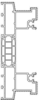
SC9K024 sup. vista mm. 230 Kg./m 3.351
