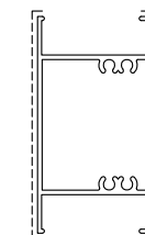
D3260230 sup.vista mm. 175 Kg./m 1.307 TAPPO L-ITES1896
