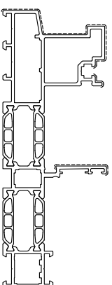
SC9K014 sup. vista mm. 180 Kg./m 3.184
