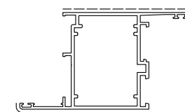
D3210289 sup.vista mm. 152 Kg./m 1.396
