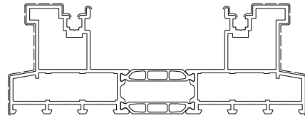
SC9K020 sup.vista mm. 000 Kg./m 3.527
