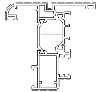
D1057011 Kg/m 1.719 Sup. in vista mm 169 TAPPO EST. D4240303 TAPPO INT. D4240304
