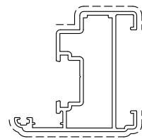
D3260021 Kg./m 0.780 sup.vista mm. 102 TAPPO D4240076
