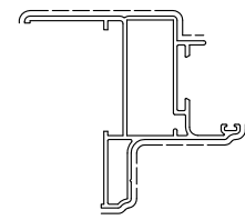
D0050027 sup.vista mm. 151 kg/m 1.121
