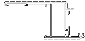
D3260036 sup.vista mm. 155 kg/m 0.992
