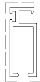
D3290161 sup.vista mm. 70 Kg./m 0.325
