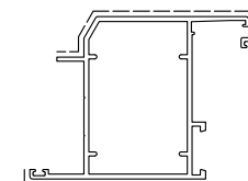
D0024463 sup.vista mm. 163 kg/m 1.336 TAPPO D0013D60
