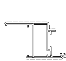
D0050025 sup.vista mm. 134 kg/m 0.905
