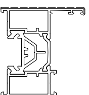
SC9V102 sup. vista mm. 116 Kg./m 1.807
