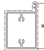
D0050036 sup.vista mm. 210 kg/m 0.888 TAPPO D00AW302 (SPORTELLO) TAPPO D00AW401 (FISSO)
