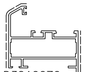
D3210070 sup.vista mm. 117 Kg/m 1.072
