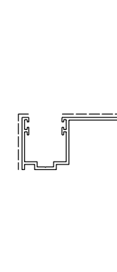
D3290111 sup.vista mm. 95 Kg./m 0.653
