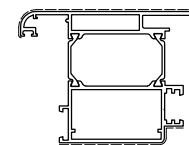
D1210885 Kg/m 2.534 Sup. in vista mm 208 TAPPO EST. D4240166 TAPPO INT. D4240304
