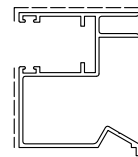
D0015127 sup.vista mm. 86 Kg./m 0.907 TAPPO D4240048
