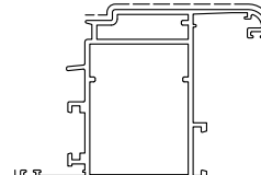
D3210292 sup.vista mm. 149 Kg./m 1.636
