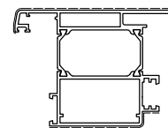
D1210883 Kg/m 2.542 Sup. in vista mm 210 TAPPO EST. D4240166 TAPPO INT. D4240304
