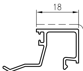
D3290103 sup.vista mm. 32.5 Kg./m 0.221
