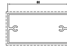
D3260226 sup.vista mm. 240 Kg./m 1.277
