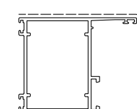
D3220070 sup.vista mm. 121 Kg./m 1.188
