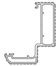
D3260268 sup.vista mm. 178 Kg./m 1.337
