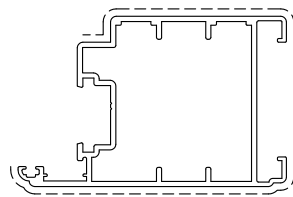
D3260020 Kg./m 1.045 sup.vista mm. 152 TAPPO D4240077
