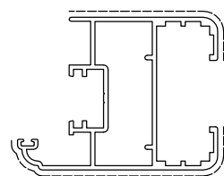
D0060104 sup.vista mm. 148 Kg./m 1.245
