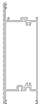
D3220071 sup.vista mm. 311 Kg./m 2.587
