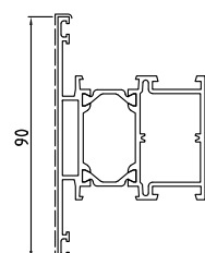
D1210462 Kg/m 1.675 Sup. in vista mm 145
