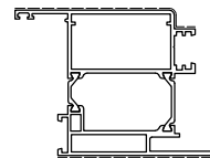
D1210887 Kg/m 2.536 Sup. in vista mm 198 TAPPO EST. D4240304 TAPPO INT. D4240166
