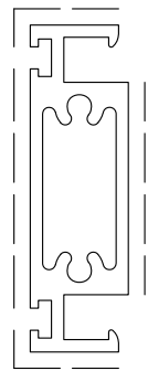
D3290162 sup.vista mm. 82 Kg./m 0.537
