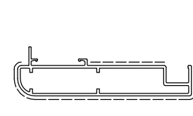
D3290112 sup.vista mm. 162 Kg./m 1.064
