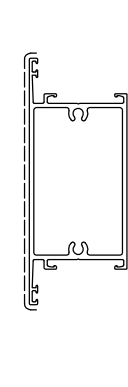
D3210269 sup.vista mm. 178 Kg./m 1.285
