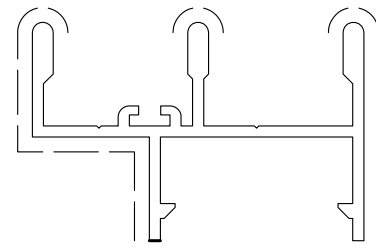
D0009179 sup.vista mm. 85 Kg./m 0.581
