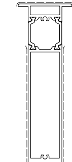
D1211027 Kg/m 2.06 Sup. in vista mm 261
