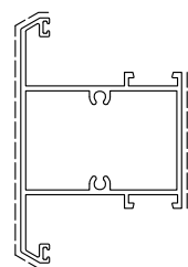
D0024462 sup.vista mm. 154 kg/m 1.496
