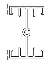
D0050005 sup.vista mm. 98 Kg./m 0.653
