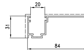
D3290160 sup.vista mm. 134.8 Kg./m 0.815
