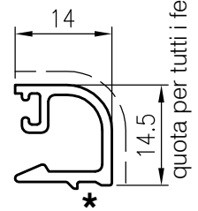
D3290109 sup.vista mm. 25.5 Kg./m 0.181
