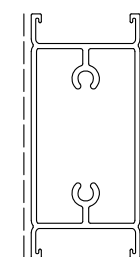
D0050106 kg/m. 0.875 Sup. in vista 134 TAPPO D00AW515 (SPORTELLO) TAPPO D00AW507 (FISSO)
