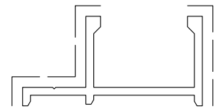
D0008713 sup.vista mm. 52 Kg./m 0.286
