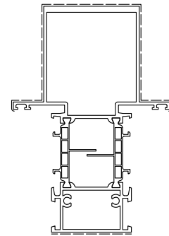
D1060057 Kg/m 2.789 Sup. in vista mm 255
