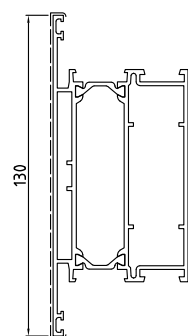
D1210464 Kg/m 2.459 Sup. in vista mm 225
