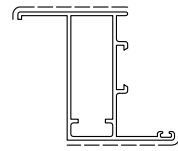
D0050002 sup.vista mm. 95 kg/m 0.845
