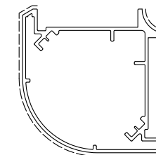
D0024499 sup.vista mm. 174 Kg./m 2.031
