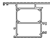
D1210881 Kg/m 2.455 Sup. in vista mm 202 TAPPO EST. D4240166 TAPPO INT. D4240304
