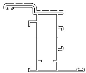
D0026214 sup.vista mm. 112 Kg./m 0.923
