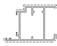
D3260239 sup.vista mm. 355 Kg./m 0.975 TAPPO L-ITES1898
