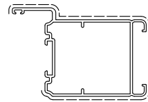
D0050028 sup.vista mm. 158 kg/m 1.015 TAPPO D00AW403 TAPPO D00AW304 (T/Z)
