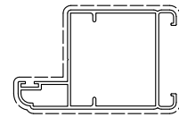
D0050044 sup.vista mm. 193 kg/m 0.948 TAPPO D00AW450
