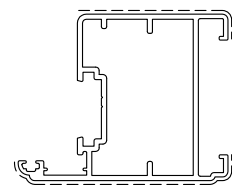
D3260257 kg/m. 0.856 sup. in vista mm. 110 TAPPO D4240152
