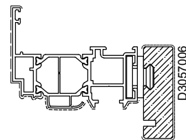
D1057046 Kg/m 1.469 Sup. in vista mm 62
