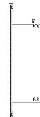
D3220020 sup.vista mm. 298 kg/m 2.014
