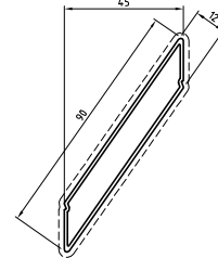
D3260225 sup.vista mm. 190 Kg./m 0.605
