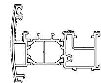
D1057048 Kg/m 1.484 Sup. in vista mm 77 TAPPO D4057014
