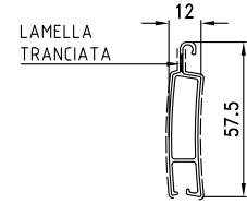
D0031D80 sup.vista mm. 117 Kg./m 0.367 TAPPO D0031D23
