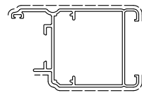
D0050026 sup.vista mm. 138 kg/m 0.986 TAPPO D00AW402 TAPPO D00AW421 (T/Z)
