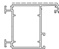
D0024461 sup.vista mm. 118 kg/m 1.372
