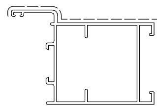
D0050008 sup.vista mm. 162 Kg./m 1.048 TAPPO D00AW043
