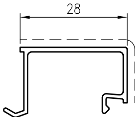
D3290106 sup.vista mm. 42 Kg./m 0.231
