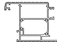
D1210889 Kg/m 2.621 Sup. in vista mm 210 TAPPO EST. D4240304 TAPPO INT. D4240166
