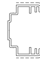
D3260054 Kg./m 0.505 sup.vista mm. 54
