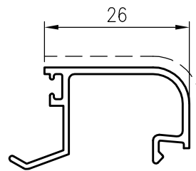
D3290108 sup.vista mm. 38 Kg./m 0.228
