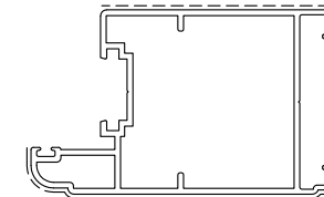
D3260262 kg/m. 1.049 sup. in vista mm.148 TAPPO D4240153
