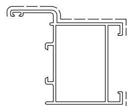
D0050003 sup.vista mm. 128 Kg./m 0.867 TAPPO D00AW042
