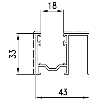
D3290159 sup.vista mm. 93 Kg./m 0.672 TAPPO D4240117
