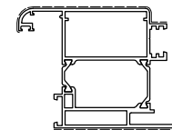
D1210891 Kg/m 2.614 Sup. in vista mm 208 TAPPO EST. D4240304 TAPPO INT. D4240166
