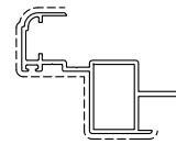
D3280020 sup.vista mm. 111 Kg./m 0.689
