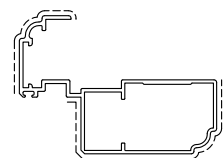
D3260172 sup.vista mm. 159 Kg./m 0.995
