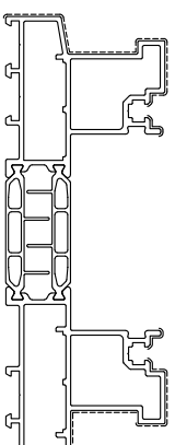
SC9K026 sup. vista mm. 312 Kg./m 3.643
