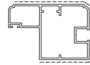
D3260201 sup.vista mm. 183 Kg./m 1.007 TAPPO D030D150
