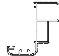
D3B 60016 sup.vista mm. 147 Kg./m 1.248
