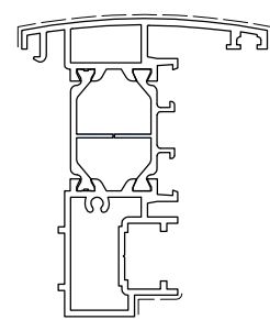
D1057021 Kg/m 1.458 Sup. in vista mm 108 TAPPO D4240302
