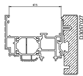
D1057046 Kg/m 1.469 Sup. in vista mm 62
