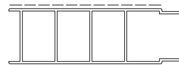
D3290132 sup.vista mm. 186 Kg./m 1.126
