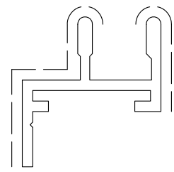
D0007592 sup.vista mm. 53 Kg./m 0.427
