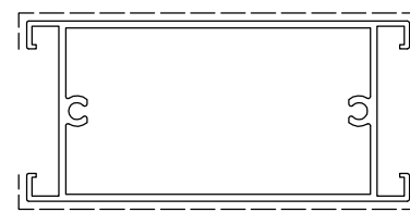
D0050039 sup.vista mm. 218 Kg./m 1.425
