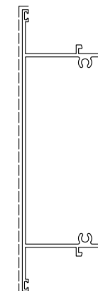
D3210086 sup.vista mm. 287 kg/m 2.036
