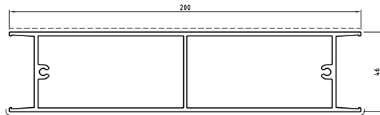
D3220091 sup.vista mm. 405 Kg./m 3.208
