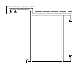
D0050021 sup.vista mm. 124 Kg./m 0.813
