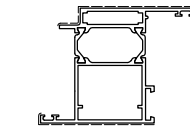
D1210901 Kg/m 1.803 Sup. in vista mm 159 TAPPO D4240266
