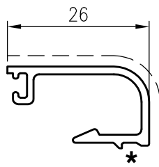
D3290110 sup.vista mm. 38 Kg./m 0.226
