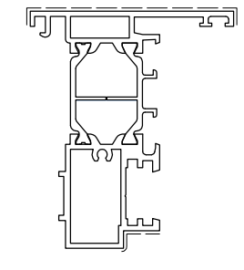
D1057016 Kg/m 1.454 Sup. in vista mm 108 TAPPO D4240300
