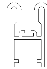
D0008712 sup.vista mm. 63 Kg./m 0.375
