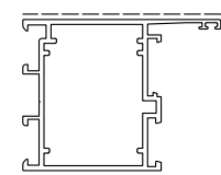
D3210290 sup.vista mm. 127 Kg./m 1.342
