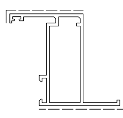
D0052217 sup.vista mm. 85 Kg./m 0.856
