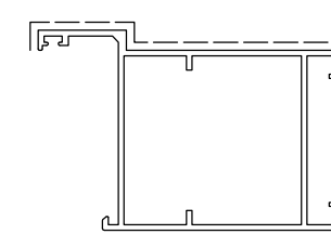
D0050020 sup.vista mm. 158 Kg./m 0.969
