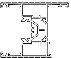
SC9V101 sup. vista mm. 169 Kg./m 2.052
