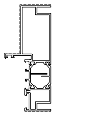
D1210871 Kg/m 2.030 Sup. in vista mm 141
