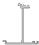
D3220073 sup.vista mm. 60 Kg./m 0.481
