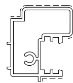
D3260259 kg/m. 0.690 sup. in vista mm. 68 TAPPO D4240146 DX TAPPO D4240147 SX
