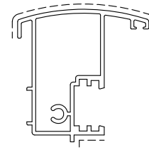
D3260027 Kg./m 0.886 sup.vista mm.77 TAPPO D4240072 DX TAPPO D4240073 SX
