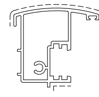
D3260023 Kg./m 0.815 sup.vista mm.72 TAPPO D4240078 DX TAPPO D4240079 SX
