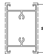
D0050043 sup.vista mm. 151 kg/m 0.988 TAPPO D00AW302 (SPORTELLO) TAPPO D00AW401 (FISSO)
