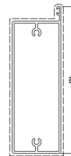
D0050033 sup.vista mm. 325 kg/m 1.588 TAPPO D00AW302 (SPORTELLO) TAPPO D00AW401 (FISSO)
