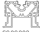
SC9C002 sup.vista mm. 000 Kg./m 1.645
