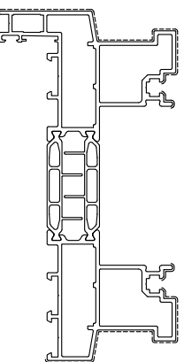
SC9K025 sup. vista mm. 248 Kg./m 3.611
