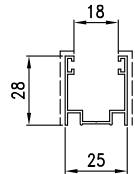
D3290155 sup.vista mm. 63.2 Kg./m 0.278
