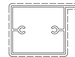
D0050006 sup.vista mm. 212 Kg./m 0.918 TAPPO D0096V88
