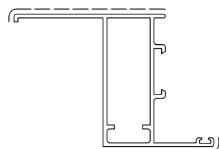
D0050023 sup.vista mm. 110 Kg./m 0.907
