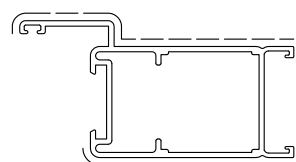
D0050102 kg/m. 0.853 Sup. in vista 179 TAPPO D00AW504
