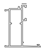
D3210307 sup.vista mm. 60 Kg./m 0.851
