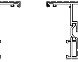
D1210904 Kg/m 2.004 Sup. in vista mm 102 TAPPO D4240266
