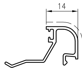
D3290107 sup.vista mm. 26 Kg./m 0.213
