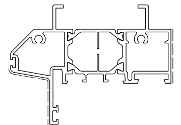
D1057041 Kg/m 1.695 Sup. in vista mm 103 TAPPO D4240117
