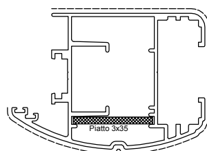
D0060059 sup.vista mm. 188 Kg./m 1.758 TAPPO DX D4B20001 TAPPO SX D4B20002
