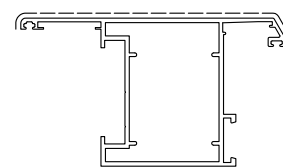
D0024471 sup.vista mm. 195 kg/m 1.587
