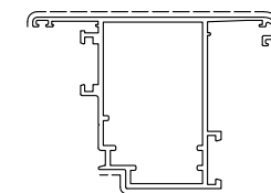
D3210302 sup.vista mm. 152 Kg./m 1.464
