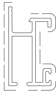
D0009182 sup.vista mm. 93 Kg./m 0.421
