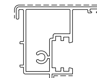
D3260265 kg/m. 0.773 sup. in vista mm. 69 TAPPO D4240150 DX TAPPO D4240151 SX
