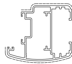
D3B60000 sup.vista mm. 158 Kg./m 1.326
