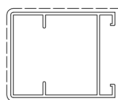
D0050009 sup.vista mm. 169 Kg./m 0.832 TAPPO D00AW043
