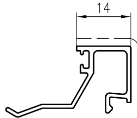
D3290102 sup.vista mm. 28.5 Kg./m 0.215
