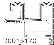
D0015170 sup.vista mm. 95 Kg/m 1.149
