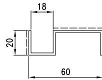
D3290147 sup.vista mm. 60 Kg./m 0.557
