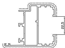
D0027492 sup.vista mm. 140 Kg./m 1.088
