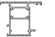
D1210902 Kg/m 1.853 Sup. in vista mm 163 TAPPO D4240266
