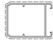
D0050031 sup.vista mm. 169 kg/m 0.805 TAPPO D00AW403
