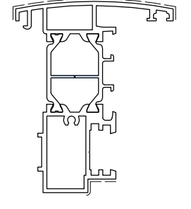
D1057017 Kg/m 1.492 Sup. in vista mm 109 TAPPO D4240301
