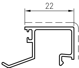
D3290104 sup.vista mm. 36.5 Kg./m 0.225
