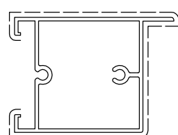
D0050024 sup.vista mm. 187 Kg./m 0.918 TAPPO D0096V89
