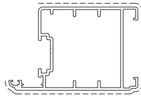
D3260015 Kg./m 0.986 sup.vista mm. 140 TAPPO D4240070
