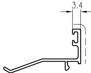
D3290100 sup.vista mm. 18 Kg./m 0.160
