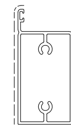
D0050107 kg/m. 0.797 Sup. in vista 114 TAPPO D00AW515 (SPORTELLO) TAPPO D00AW507 (FISSO)
