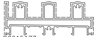
D0015177 sup.vista mm. 30 Kg/m 2.764
