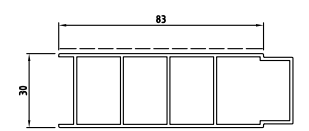
D3290132 sup.vista mm. 186 kg/m 1.126
