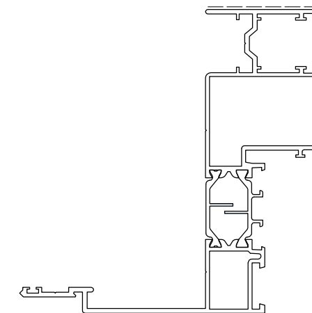
D1057023 Kg/m 2.311 Sup. in vista mm 175 TAPPO D4240117
