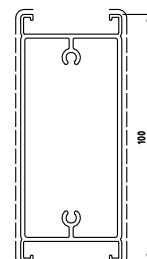
D0050032 sup.vista mm. 219 kg/m 1.420 TAPPO D00AW302 (SPORTELLO) TAPPO D00AW401 (FISSO)
