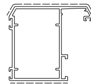
D0024473 sup.vista mm. 126 kg/m 1.266
