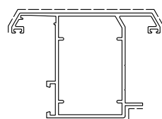
D0024464 sup.vista mm. 163 kg/m 1.401 TAPPO D0013D60
