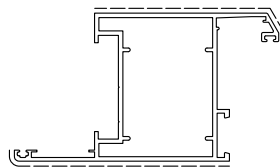
D0024470 sup.vista mm. 195 kg/m 1.587
