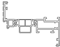
D1211284 Kg/m 1.130 Sup. in vista mm 89
