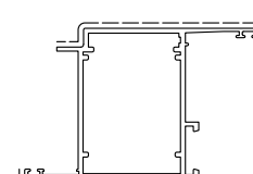
D3220068 sup.vista mm. 152 Kg./m 1.272 TAPPO D0015D30
