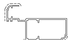
D3260044 sup.vista mm. 120 Kg./m 0.972
