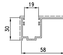
D3290111 sup.vista mm. 98 Kg./m 0.653
