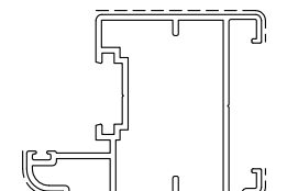
D3260261 kg/m. 0.928 sup. in vista mm. 116 TAPPO D4240153
