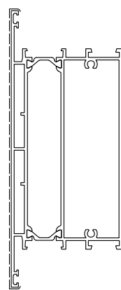
D1210461 Kg/m 3.2 Sup. in vista mm 285
