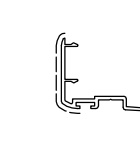
D0026261 sup.vista mm. 35 Kg./m 0.305
