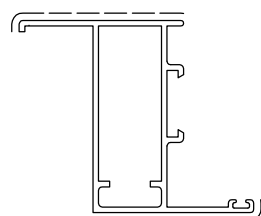
D0050002 sup.vista mm. 95 Kg./m 0.845
