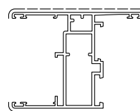
D3210299 sup.vista mm. 136 Kg./m 1.256
