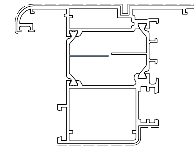
D1057015 Kg/m 2.161 Sup. in vista mm 212 TAPPO EST. D4240303 TAPPO INT. D4240304
