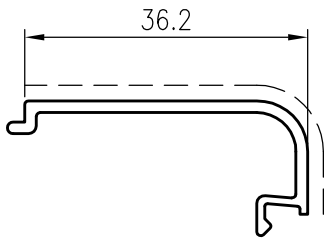
D3290123 sup.vista mm. 48 Kg./m 0.233
