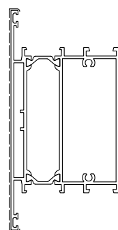
D1210460 Kg/m 2.609 Sup. in vista mm 225
