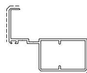
D3260234 sup.vista mm. 80 Kg./m 0.791
