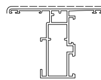
D3210300 sup.vista mm. 109 Kg./m 1.137
