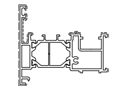
D1057049 Kg/m 1.448 Sup. in vista mm 77 TAPPO D4057014
