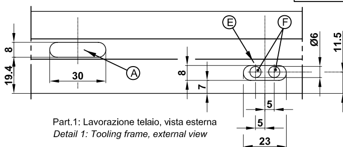
Part.1: Lavorazione telaio, vista esterna Detail 1: Tooling frame, external view
